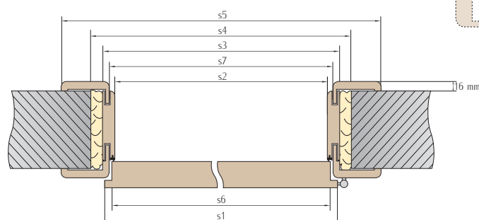
Schemat ościeżnicy regulowanej
