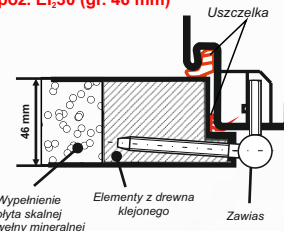
PRZEKRÓJ SKRZYDŁA - P.poż. EI,30 (gr. 46 mm)
