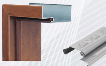
Ościeżnica KMT 15CP + próg P15
