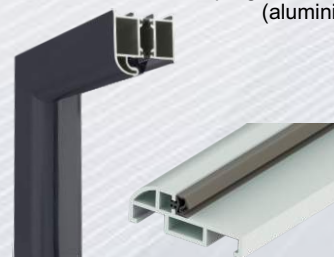
Ościeżnica ENERGY 60 + próg ENERGY 60 (aluminiowa)
